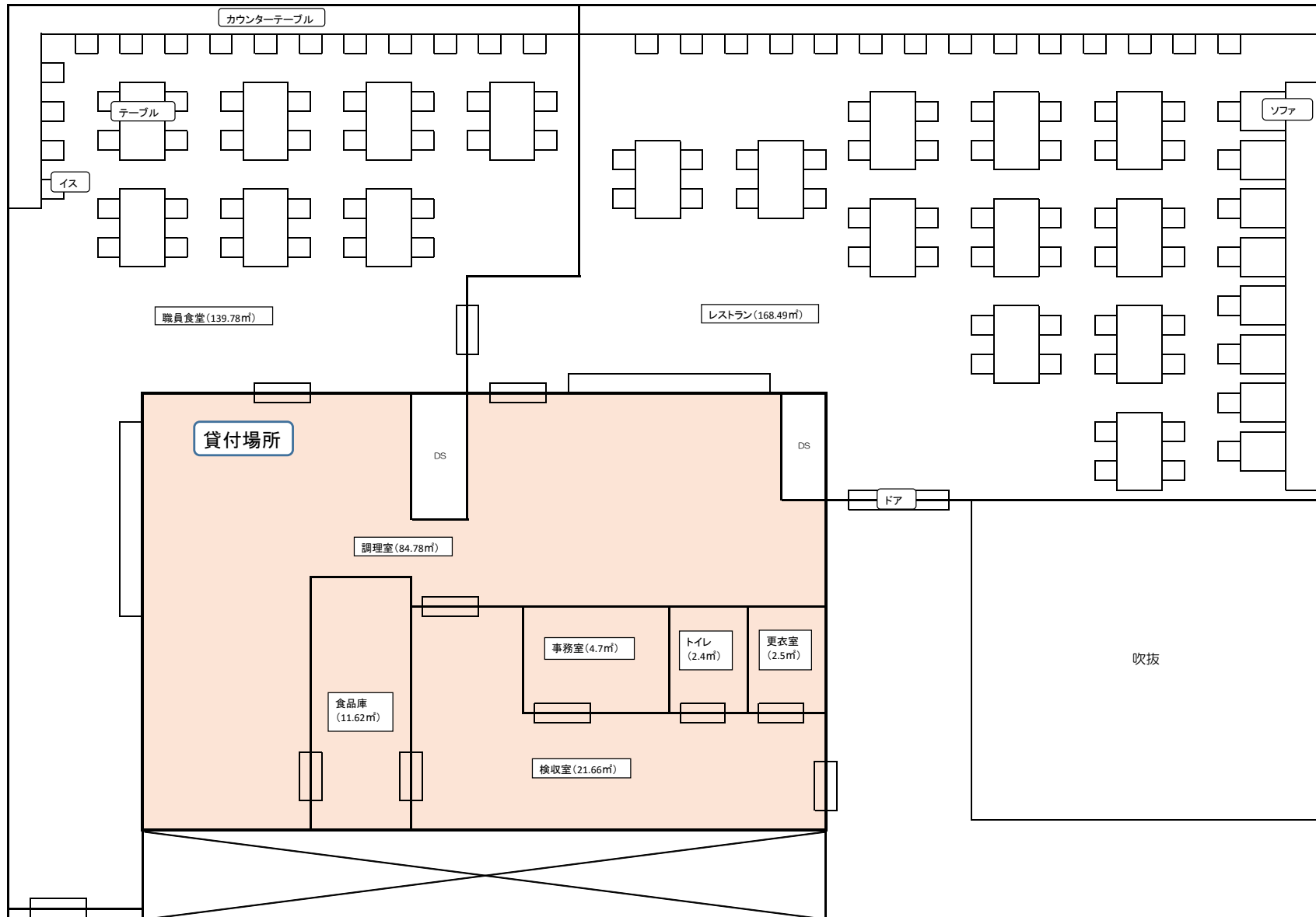
レストラン・職員食堂レイアウト（イメージ）
