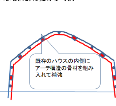
二重アーチによる補強の参考例
