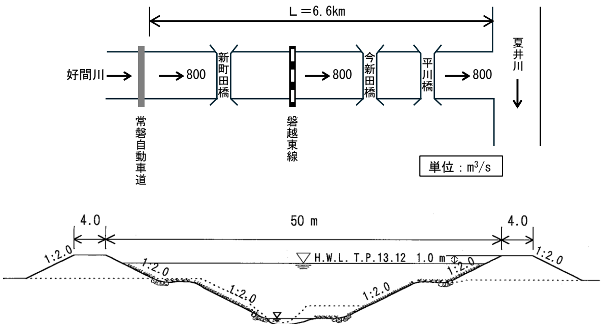
流 量 配 分 図
