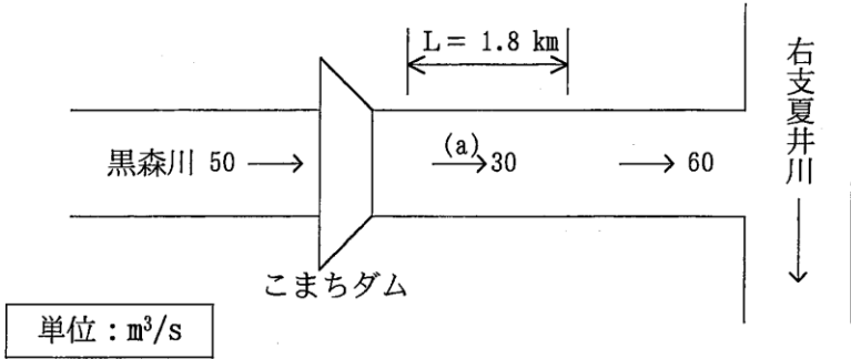
流量配分図
