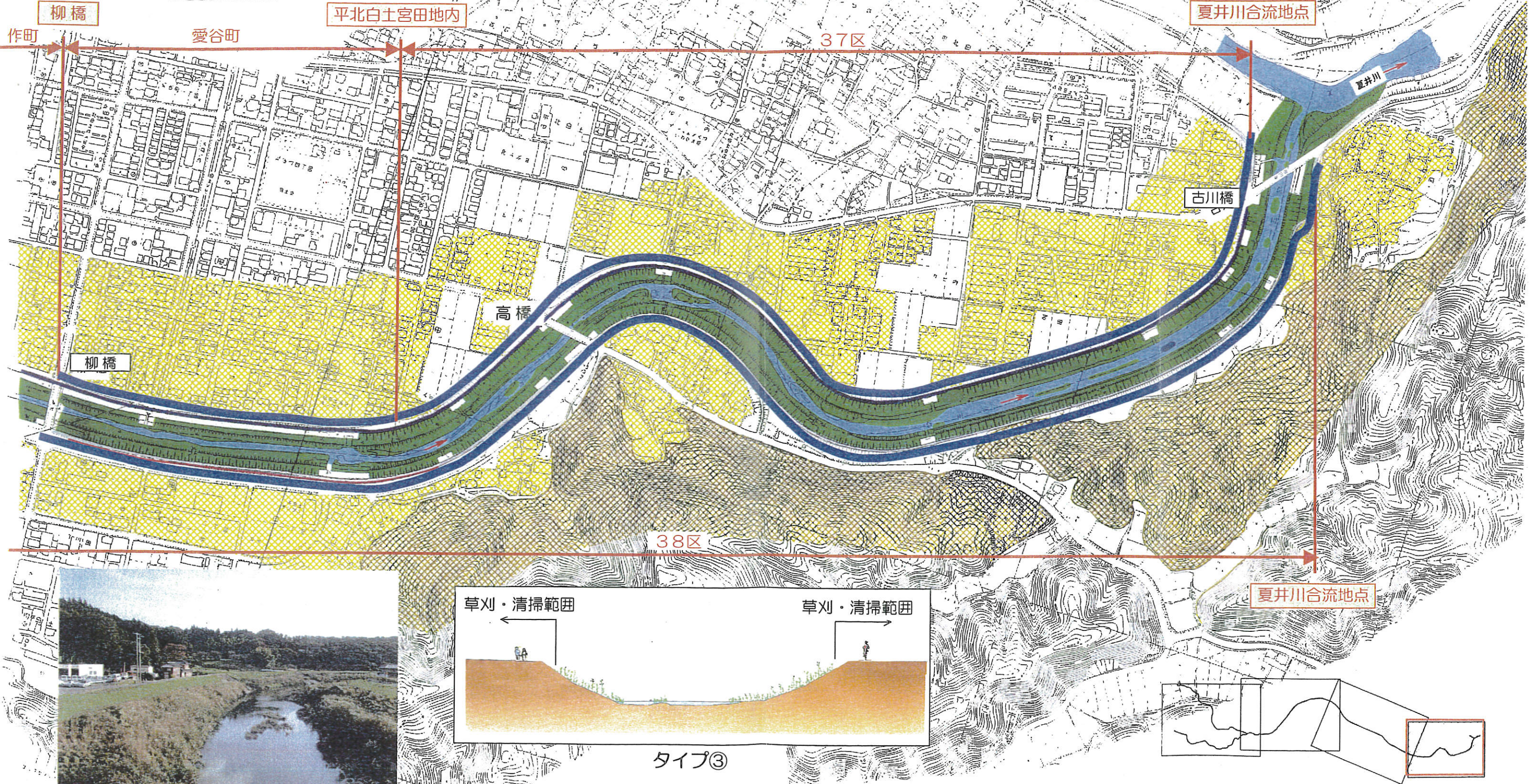
図-2.10(1) 担当区分詳細図 (生態系保全ゾーン)
