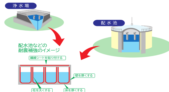
水道施設の耐震化イメージ
