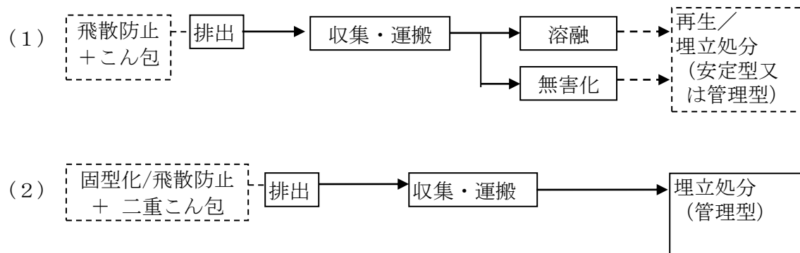
図2-2 廃石綿等の処理経路の例
