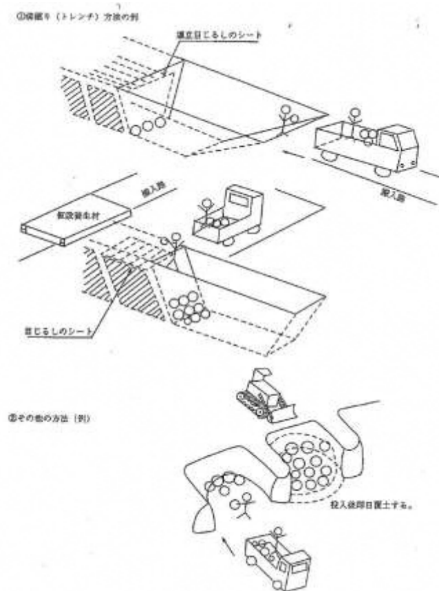
図 6-5 廃石綿等の埋立方法の例
