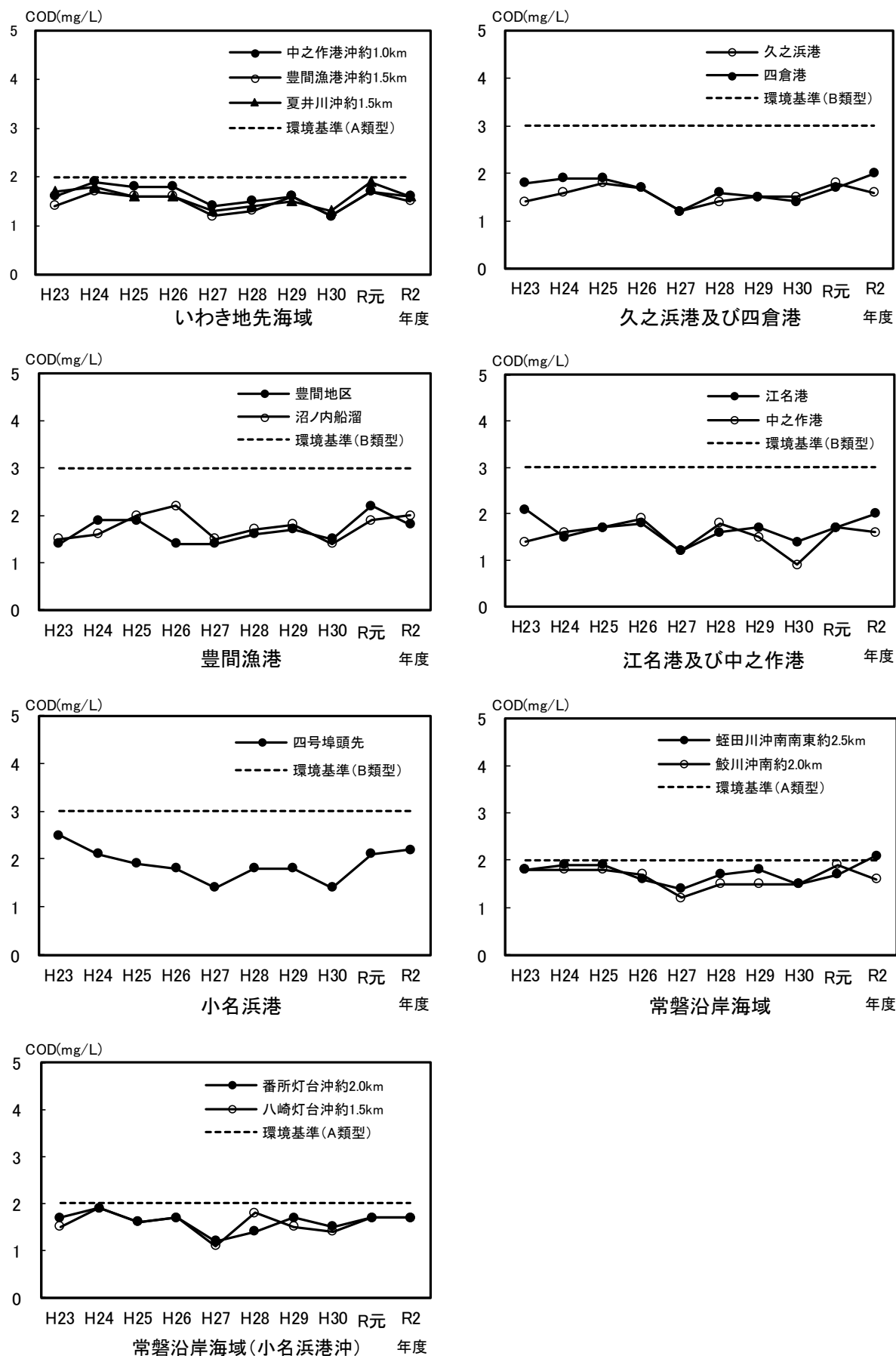
図6-3(2)-1 海域のCOD(75%水質値)経年変化
