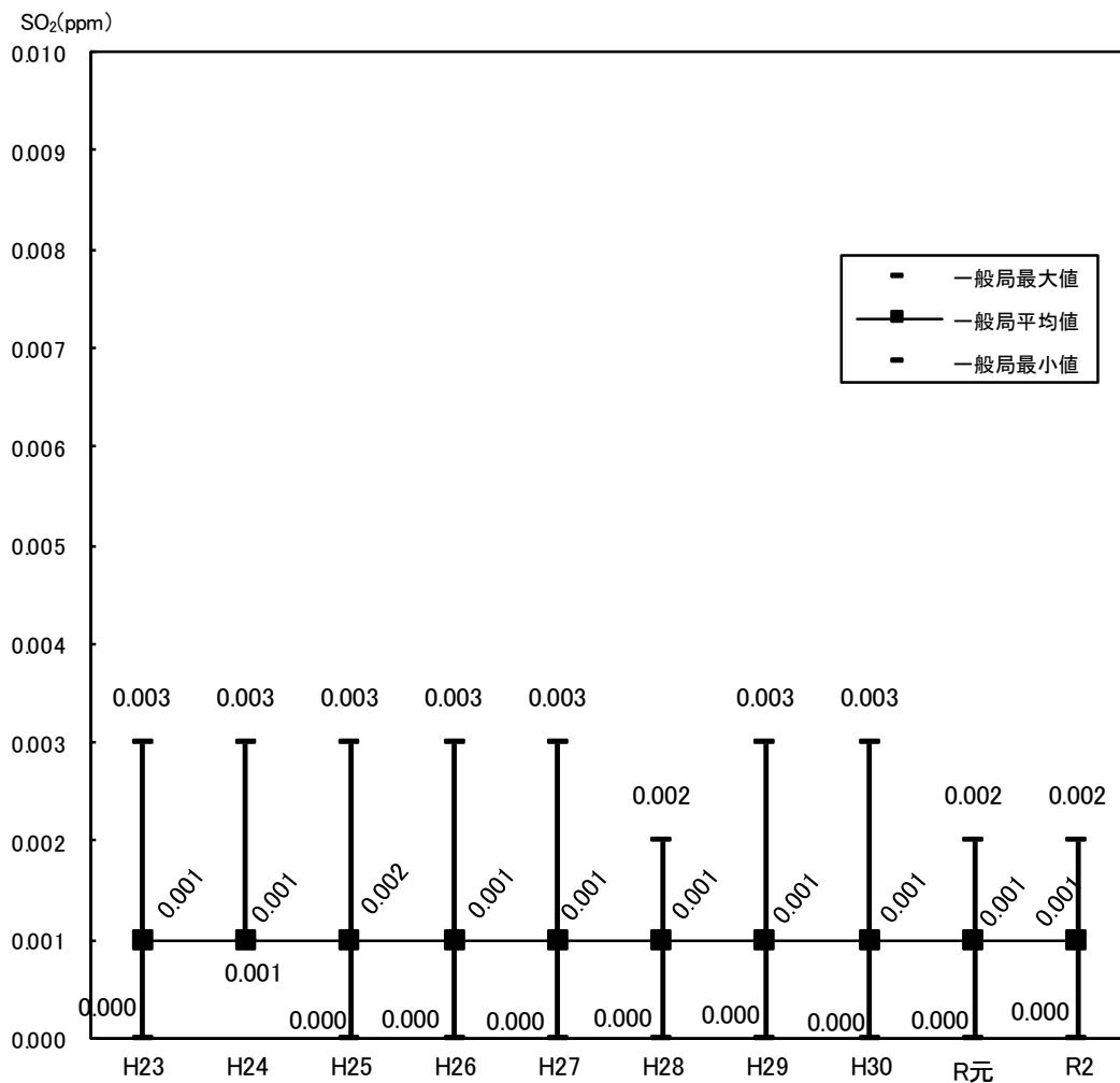
図3-3(1) 二酸化硫黄の年平均値の推移
