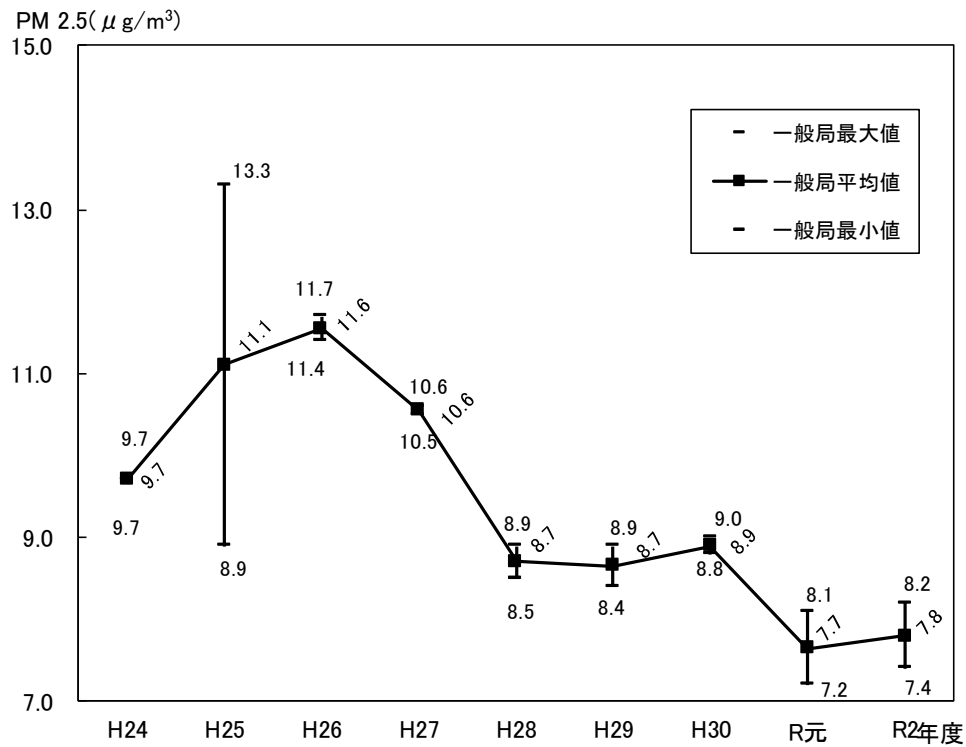
図3-3(4) 微小粒子状物質の年平均値の推移
