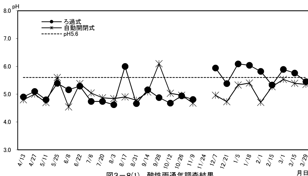
図3-8(1) 酸性雨通年調査結果
