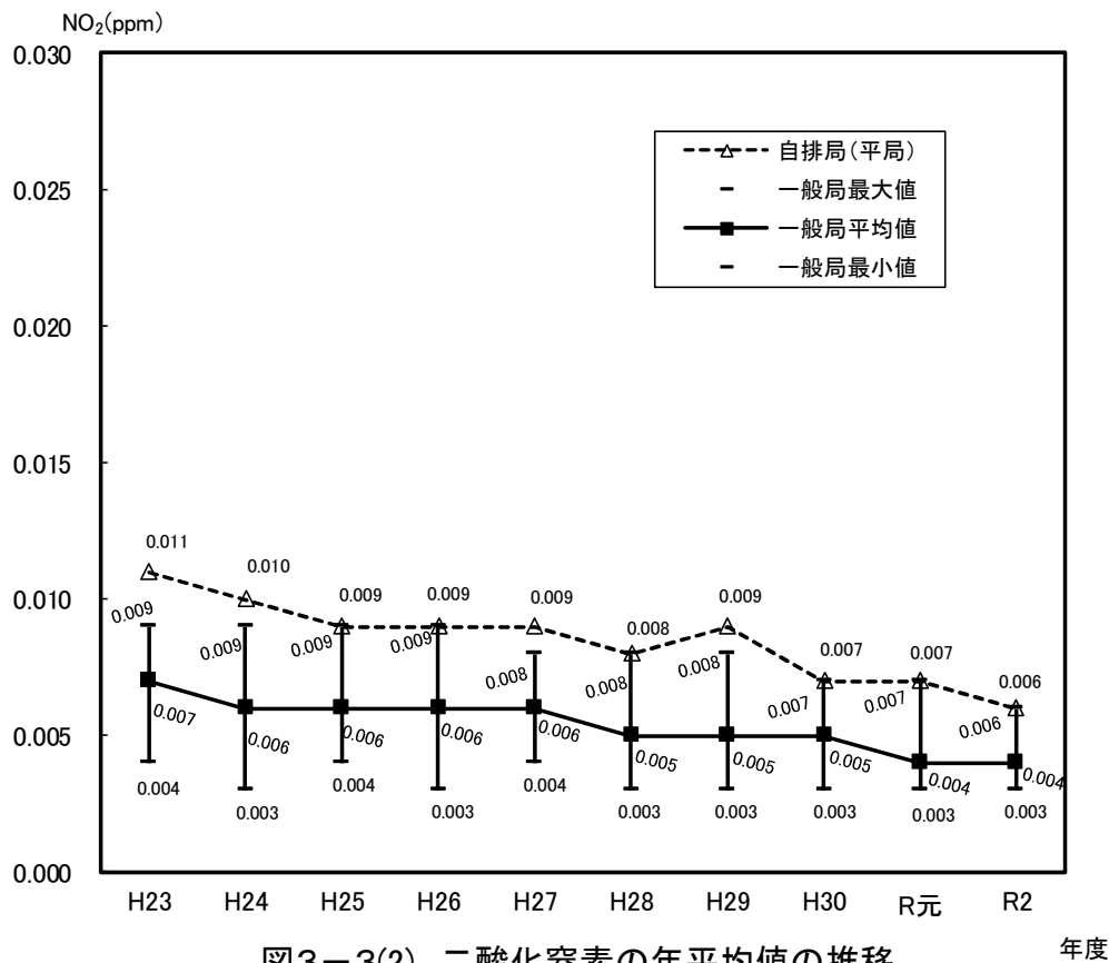
図3-3(2) 二酸化窒素の年平均値の推移
