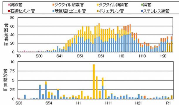
図 管路の布設年度別延長(上:上水道、下:簡易水道)
