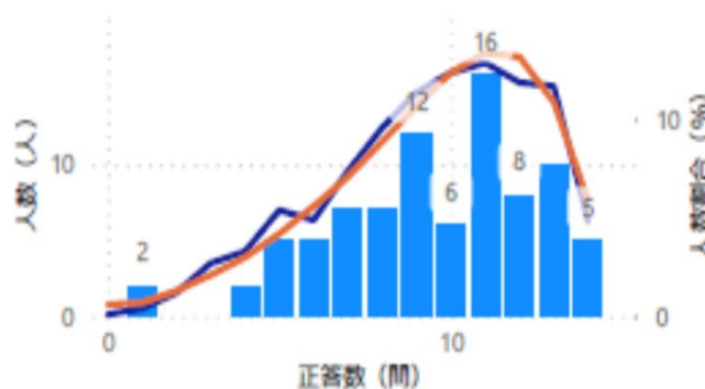
国語正答数の分布
