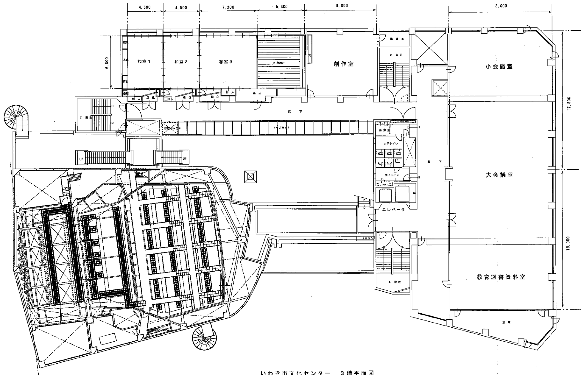
いわき市文化センター 3階平面図
