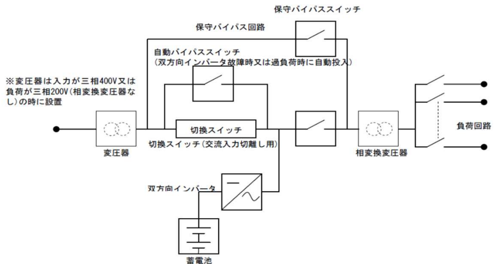
図－5.4.2.2 常時商用給電方式システム構成の参考例
