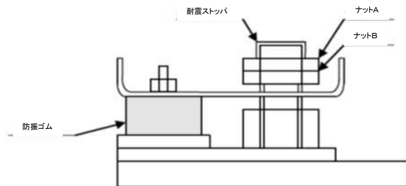
図－3.2.2 防振支持機器例 (水道施設耐震工法指針・解説 2022年版 日本水道協会)
