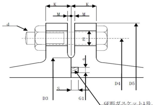
図-4.8.11 R F形(大平面座形)-G F形(溝形)フランジ メタルタッチの場合
