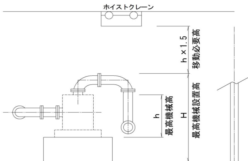
図 1 ホイストクレーン設置高
