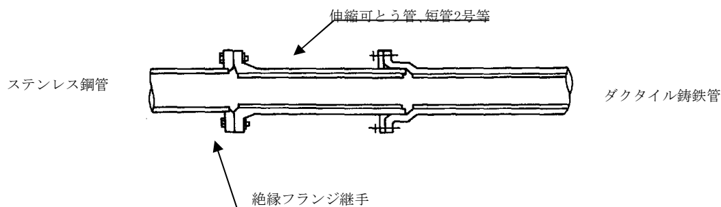
図2 異種金属管の接続 (ダクティル鋳鉄管とステンレス鋼管との接続法)
