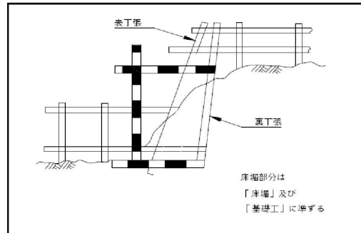
切取り法面
