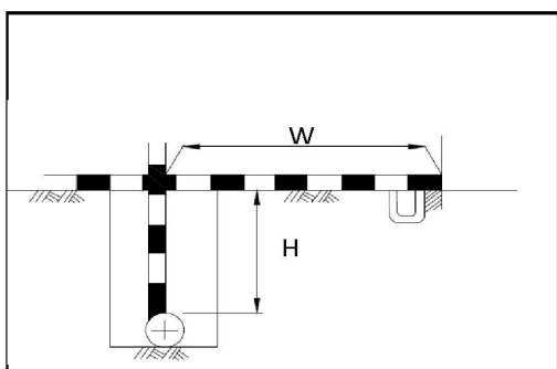
布設位置
