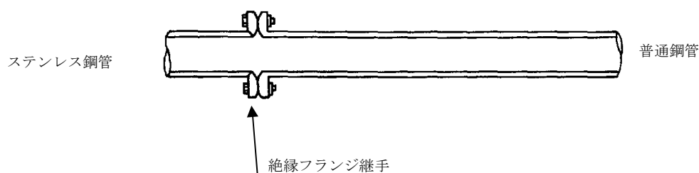
(普通鋼管とステンレス鋼管との接続法)
