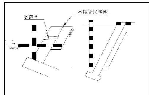
石 積
