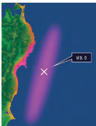
■図1-1 東北地方太平洋沖地震の震源地、地震発生地帯、津波到達点
