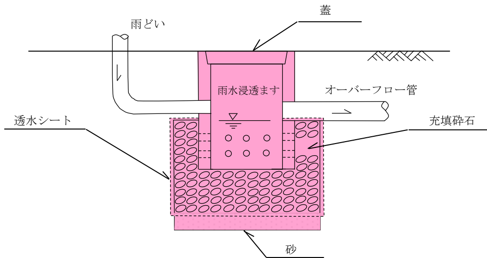
断面図
