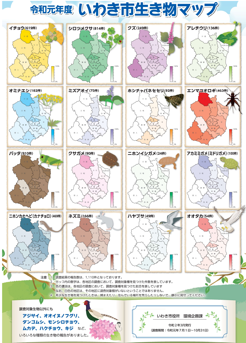
図 5-4-12 野生生物生息生育育成調査の結果
